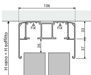
tipologia 2S doppio binario a soffitto
