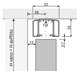
tipologia 1SRB binario monorotaia a soffitto pannello raso binario
