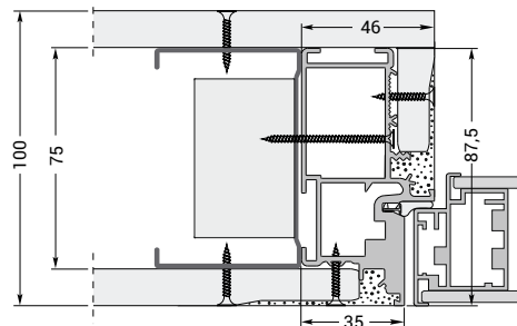
TELAIO SU PARETI CARTONGESSO con una lastra spessore parete finita 100 mm
