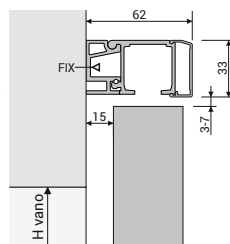
tipologia 1PRB-bat binario monorotaia a parete con battiscopa pannello raso binario
