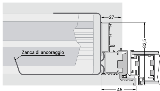
TELAIO SU PARETI INTONACO
