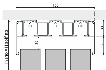
tipologia 3S triplo binario a soffitto
