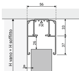
tipologia 1S binario monorotaia a soffitto
