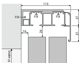
tipologia 2P doppio binario a parete
