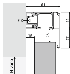
tipologia 1P-bat binario monorotaia a parete con battiscopa
