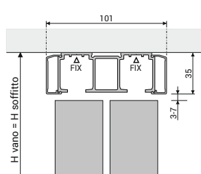
tipologia 2SRB doppio binario a soffitto pannello raso binario
