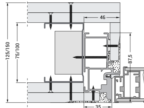
TELAIO SU PARETI CARTONGESSO con due lastre spessore parete finita 125/150 mm
