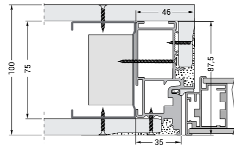
TELAIO SU PARETI CARTONGESSO con una lastra spessore parete finita 100 mm
