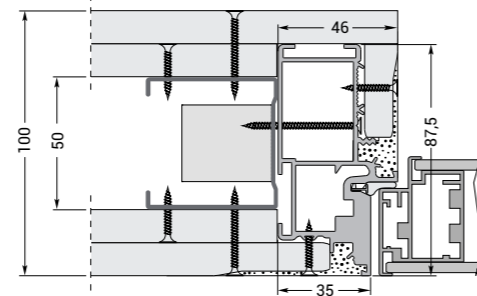
TELAIO SU PARETI CARTONGESSO con due lastre spessore parete finita 100 mm
