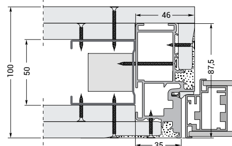
TELAIO SU PARETI CARTONGESSO con due lastre spessore parete finita 100 mm
