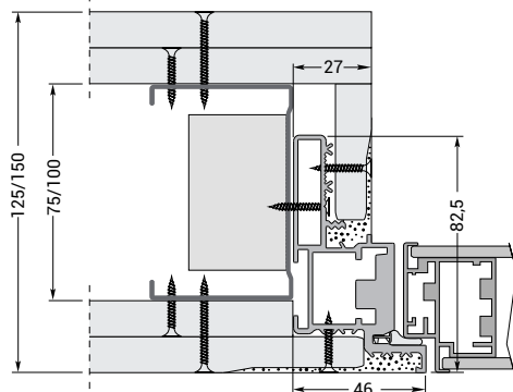
TELAIO SU PARETI CARTONGESSO con due lastre spessore parete finita 125/150 mm
