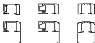
SCORRIMENTO AD 1 VIA
