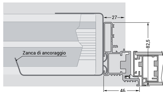
TELAIO SU PARETI CARTONGESSO con una lastra spessore parete finita 100 mm
